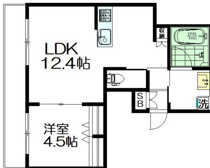
【間取り図】
